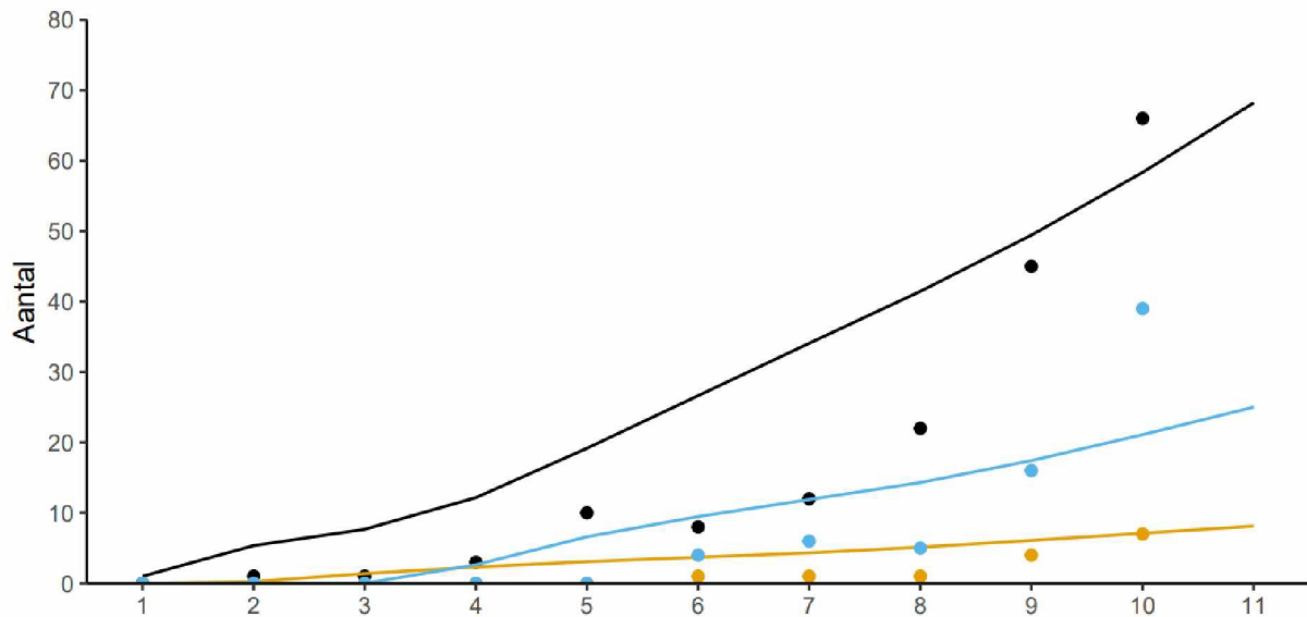
Figuur 7. 32 Ontwikkeling van de populatie wolven in Nederland volgens veldgegevens (punten) en volgens het scenario dat de vestigingskans 90% bedraagt (lijnen). Zwart: aantal wolven, blauw: aantal welpen, oranje: aantal roedels. Modeljaar 1 is gelijkgesteld aan de velddata van 2014 et cetera.
