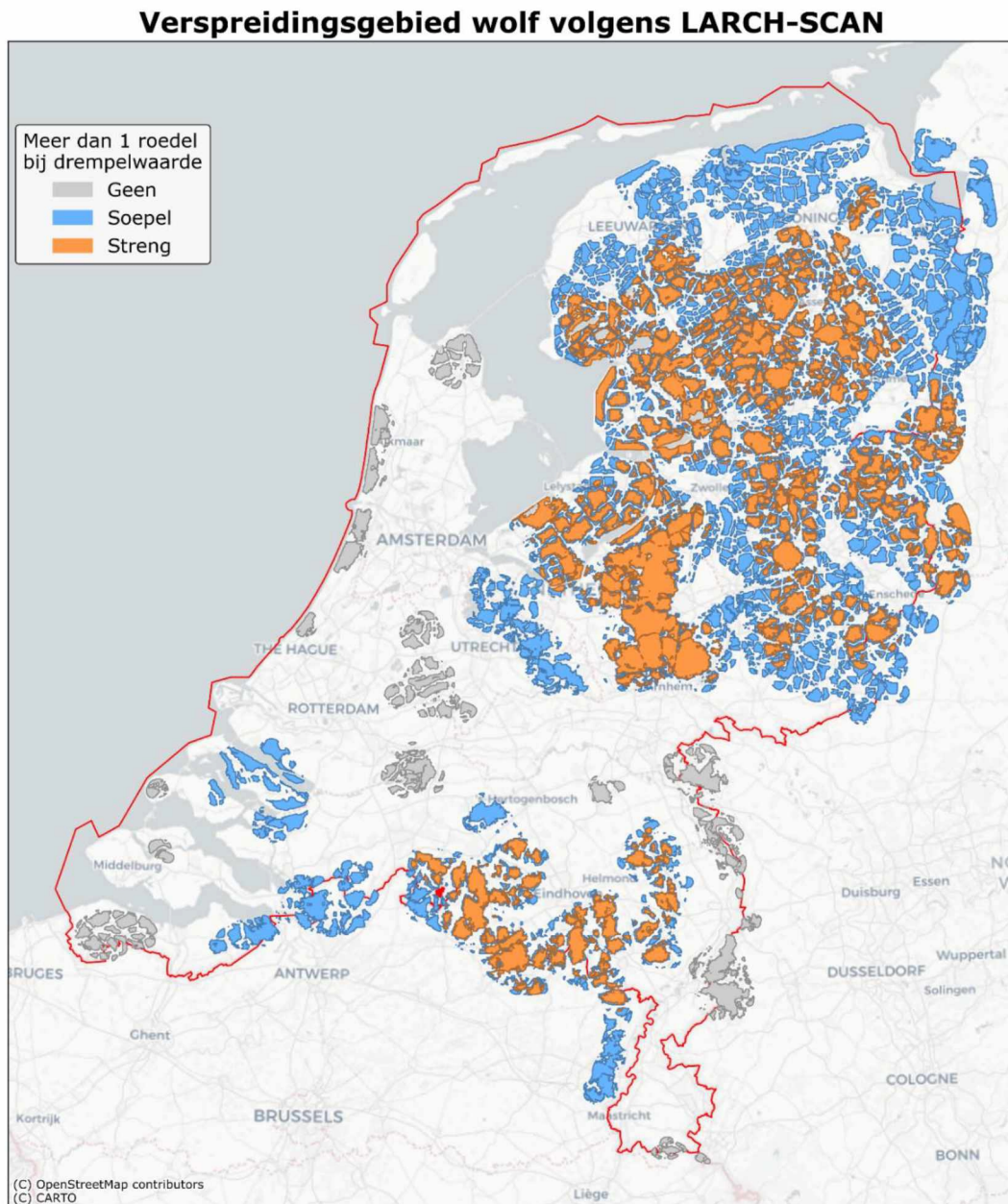
Figuur 4. 25 Potentieel verspreidingsgebied van de wolf in Nederland volgens het model 'LARCH-SCAN'. De blauwe en oranje gebieden zijn bij respectievelijk de lage en de hoge drempelwaarde minstens één roedel groot. De grijze gebieden zijn kleiner dan één roedel en alleen aangewezen bij de lage drempelwaarde.
