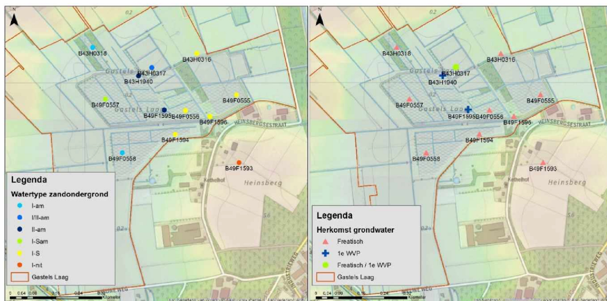
Figuur 3-17: Grondwaterkarakteristieken (links) en herkomst grondwater (rechts) in het freatisch pakket onder Gastels Laag en de Heinsberg ( 5.1.2.e 2022). Zie Tabel 3-5
