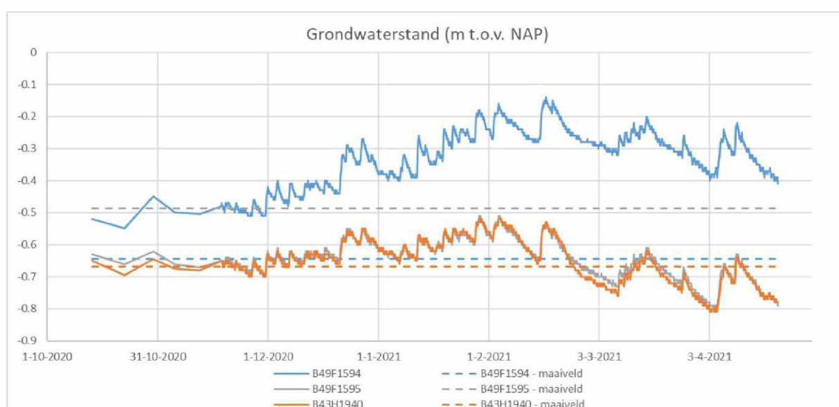
Figuur 3-16: Grondwaterstand in meter ten opzichte van NAP in de peilbuizen van het meetnet van Brabant Water die in het Gastels Laag liggen en de maaiveld hoogte van deze peilbuizen (stippellijn).
