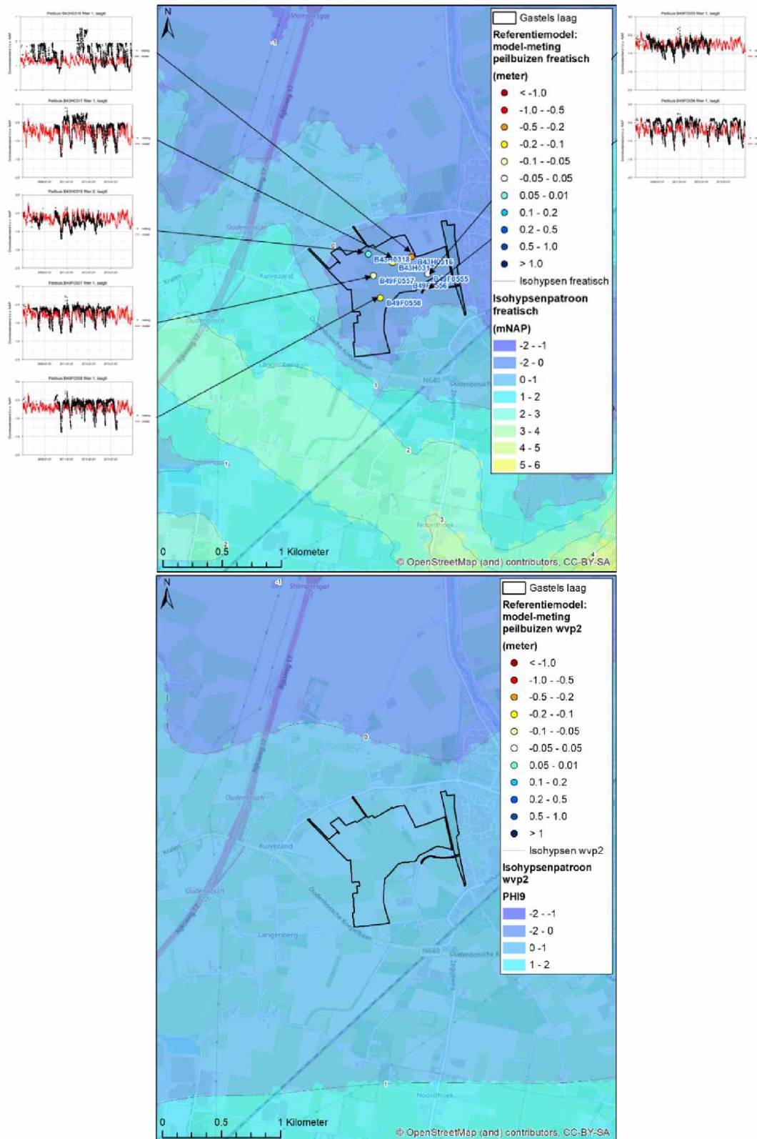
Figuur 5-1: Isohyspenpatroon in het eerste Watervoerende pakket (boven) en tweede watervoerende pakket. De punten tonen de locaties van de peilbuizen waarmee het model is geverifieerd. De kleur van het punt geeft aan hoeveel berekening en meting verschillen (in meters). De grafieken naast de kaart tonen de verschillen tussen model en meting voor de peilbuizen in het watervoerende pakket, de rode lijn zijn gemodelleerde grondwaterstanden en de zwarte punten zijn de gemeten grondwaterstanden.
