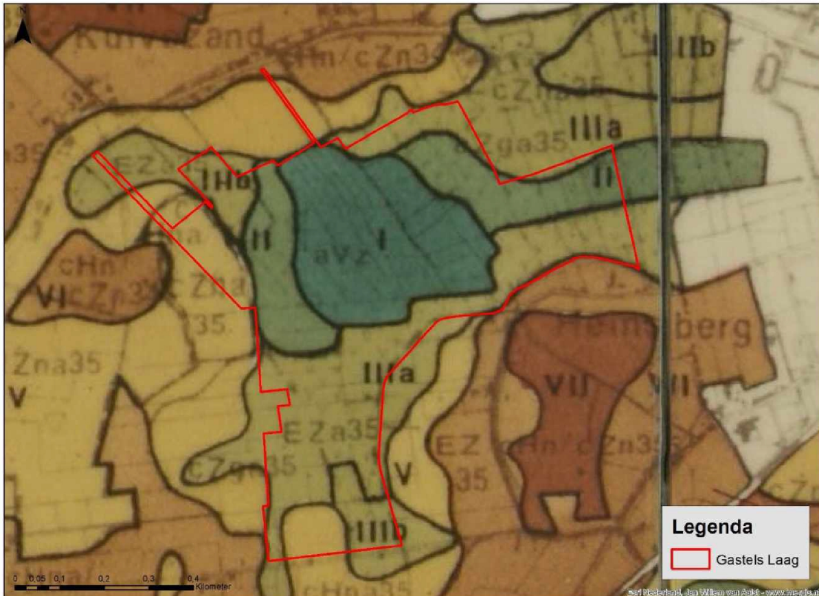
Figuur 3-9: Grondwatertrappenkaart (1:25.000) uit 1972 gemaakt ter voorbereiding van de Ruilverkaveling Oud Gastel – Oudenbosch (5.1.2.e). De lage madeveengronden (aVz) hebben een Gt I of Gt II. De hogere beekoordgronden (cZga35) hebben binnen Gastels Laag een Gt II of Gt IIIa.
