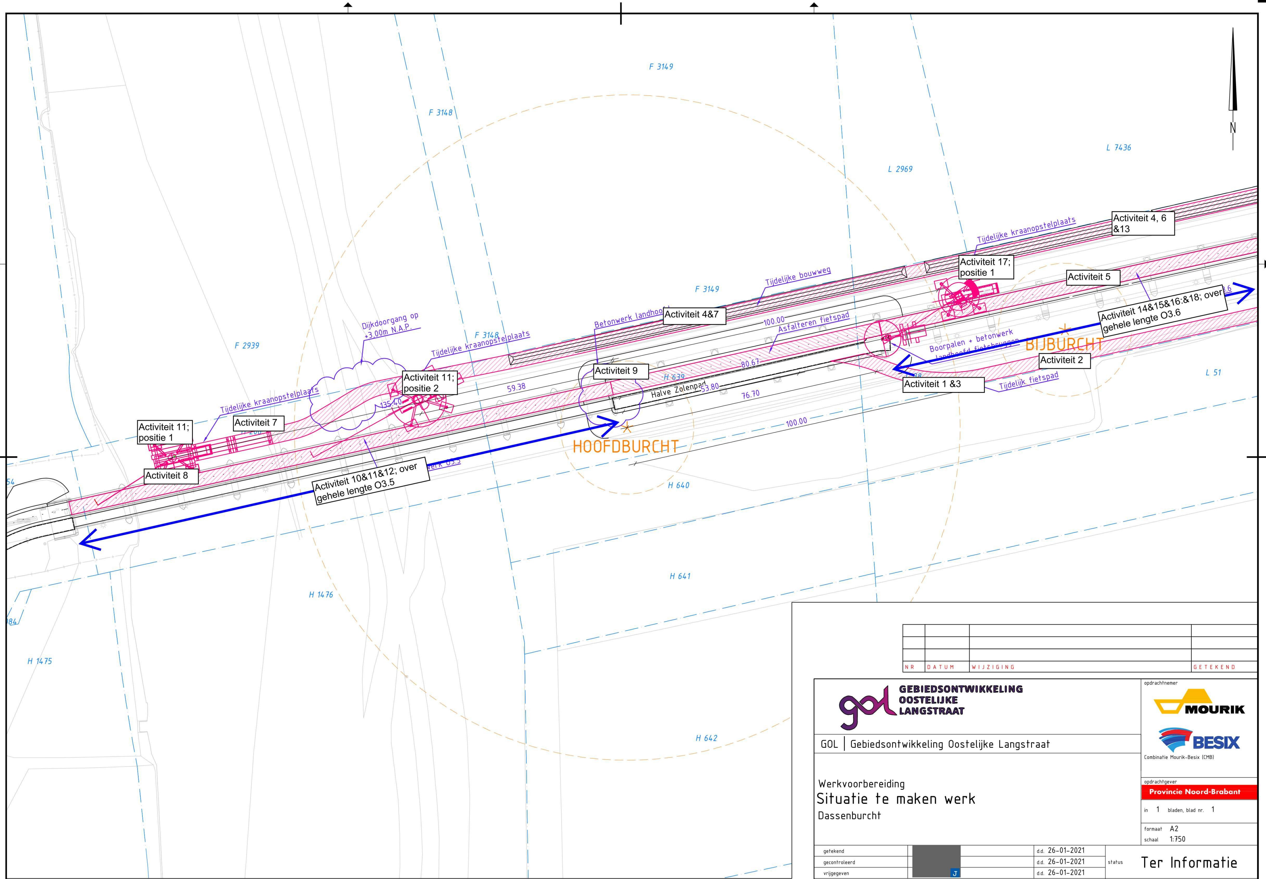
Situatieoverzicht 1:750
