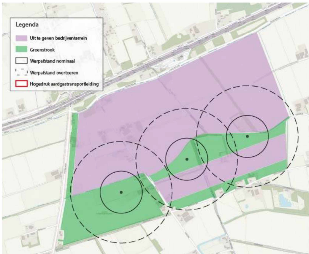
Figuur 6.6 Werpafstand bij nominaal toerental en werpafstand bij overtoeren voorkeursalternatief
