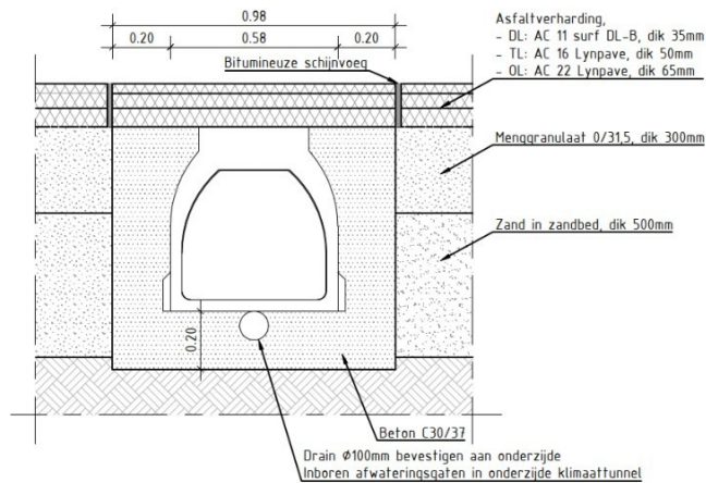
Afbeelding 18. Voorbeeld Aco Pro klimaattunnel.
